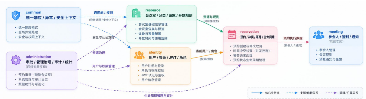
图 2-2 后端 Domain 模块依赖图
